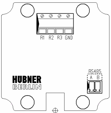
Bild 19: Belegung Klemmenkasten DSL.R
