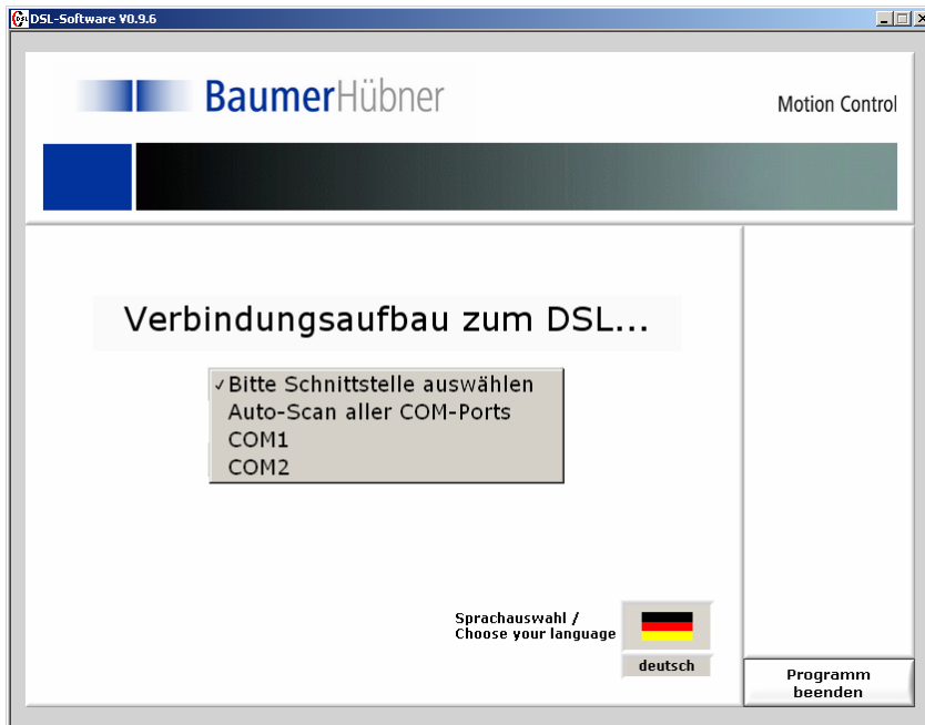
Bild 5: Auswahl COM-Port
