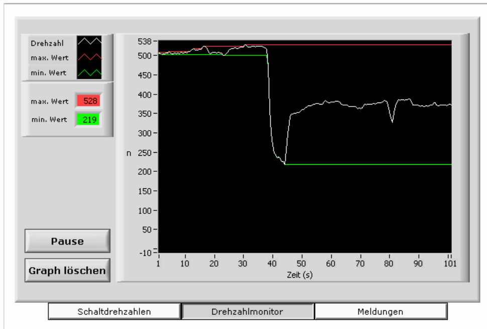
Bild 12: Register Drehzahlmonitor
