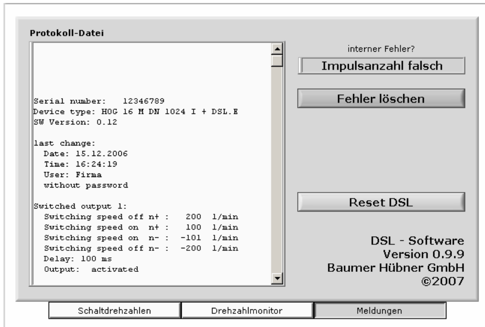
Bild 13: Register Meldungen
