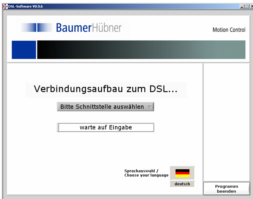
Bild 4: Startbildschirm
